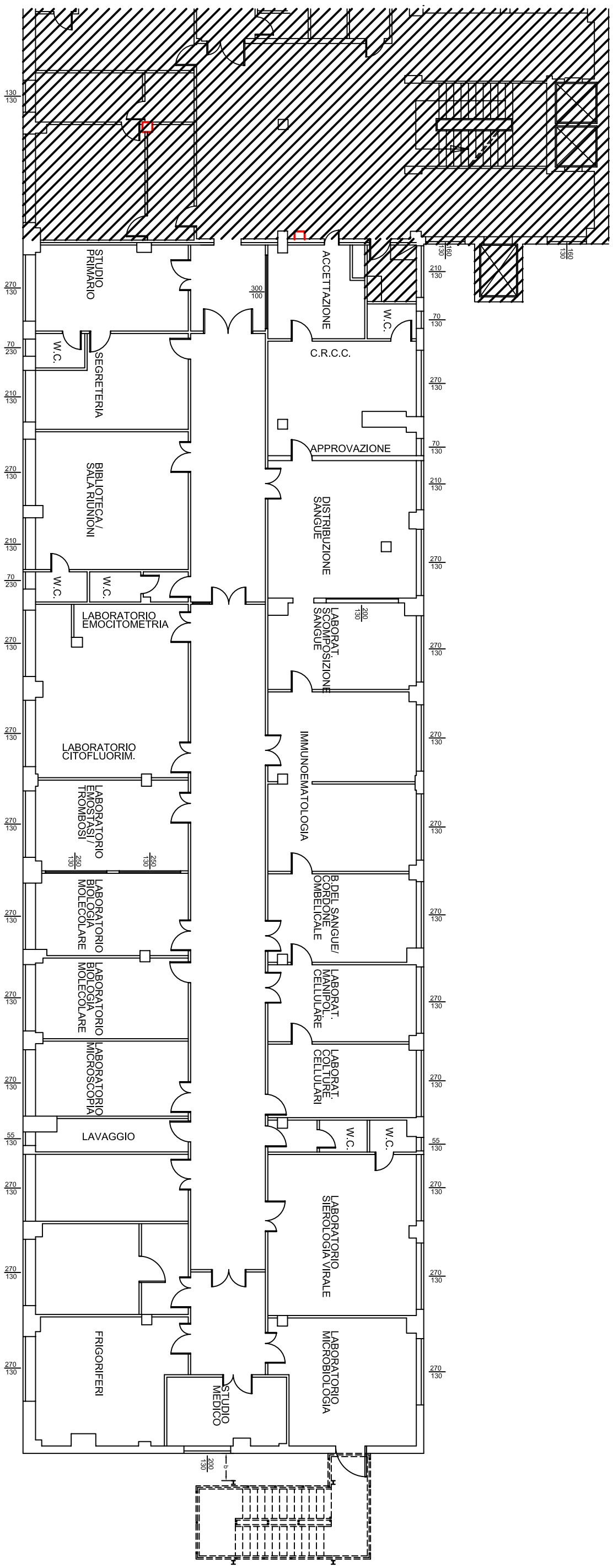
PLANIMETRIA DELL'U.O. AL PIANO SECONDO scala 1:100
